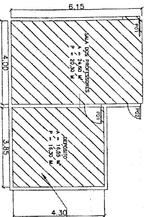
PLANTA BAIXA - FORRO DE SALAS
