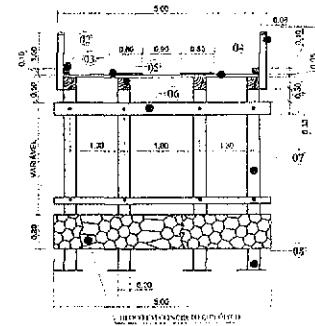
SEÇÃO TRANSVERSAL - PILARES DE CABECEIRA
