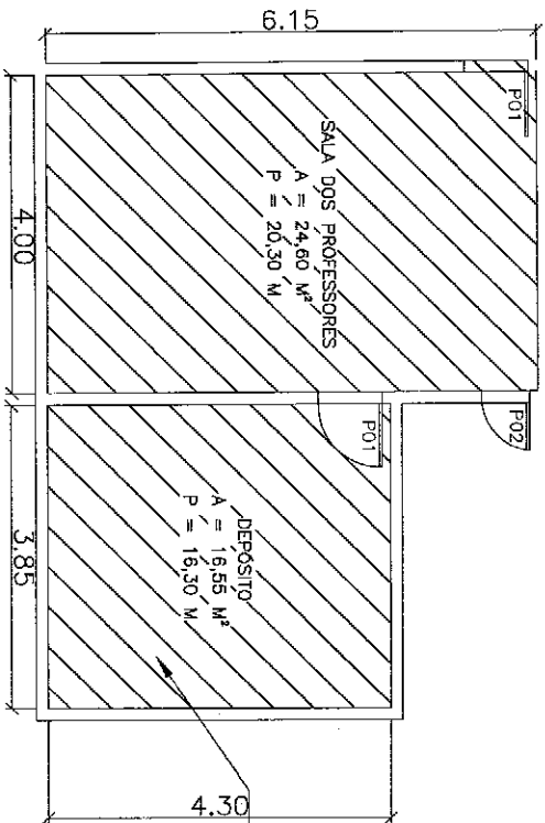
PLANTA BAIXA - FORRO DE SALAS
