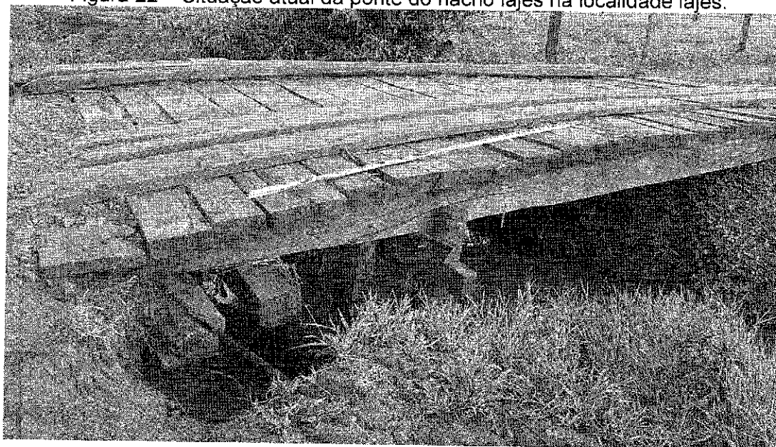
Figura 22 – Situação atual da ponte do riacho lajes na localidade lajes.
