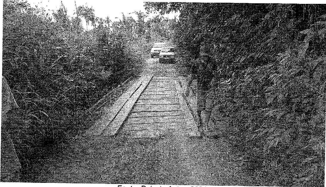
Figura 19 – Situação atual da ponte do riacho fundo na localidade nova Veneza.
