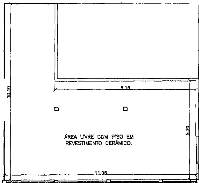
PLANTA BAIXA DA ÁREA LIVRE
